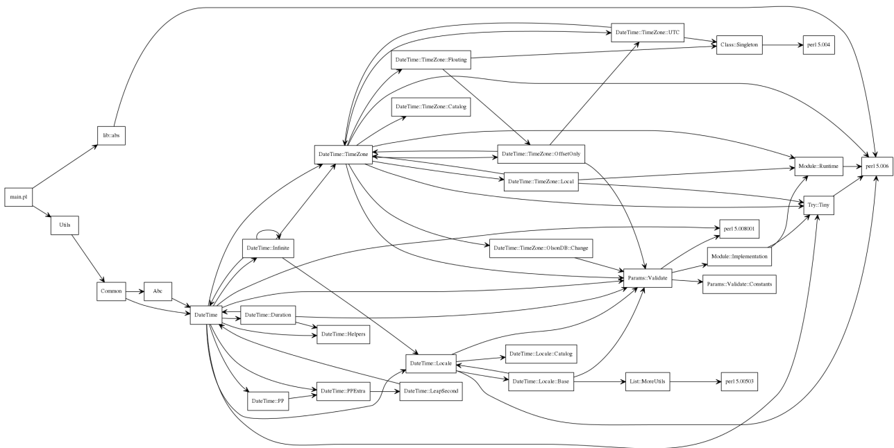
Рис. 1: Граф зависимостей
